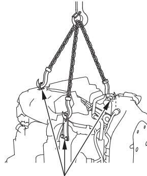
ПОДЪЕМНЫЕ ПРОУШИНЫ (3)
